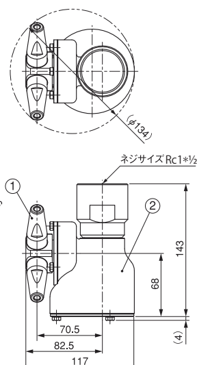
①ノズル ②本体
